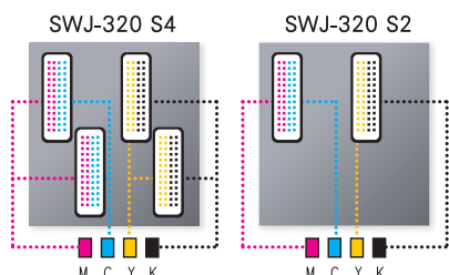
噴頭配置示意圖
